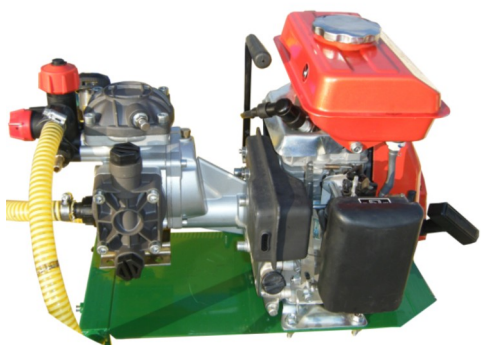
DETALLE BOMBA CON MOTOR
